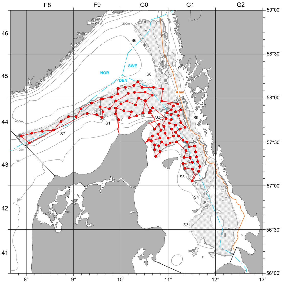
Figur 1. Stationskort UWTV Monitoring 2020: Danmark i strata 1, 2, 5, 7 and 8 med RV Havfisken (103 stations in alt deraf 2 stationer taget to gange), de andre strata dækkes af Sverige).
