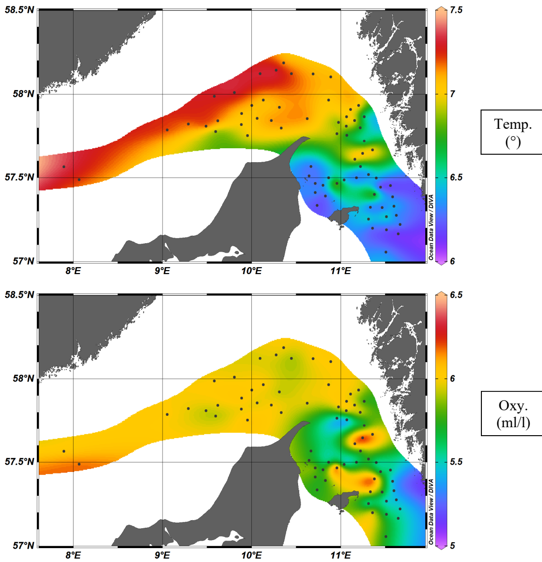
Figur 3. Temperatur (°) og ilt (ml/l) ved bunden, UWTV Monitoring 2020 Danmark.
